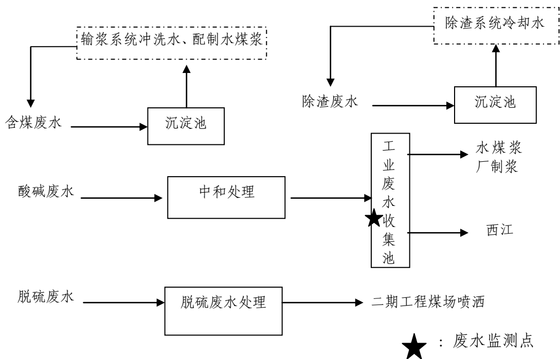
废水处理流程图
